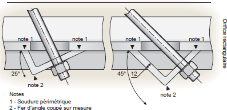
Détail C : Attache de terminaison de la barrière de grillage renforcée
