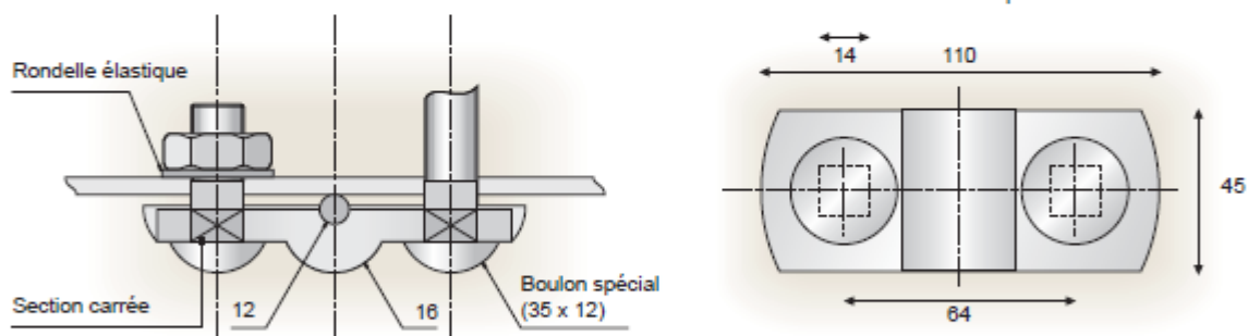
Détail B : U double en fer (120 mm)
