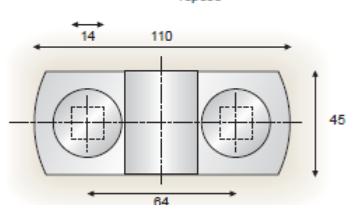
Détail C : Attache de terminaison de la barrière de grillage renforcée
